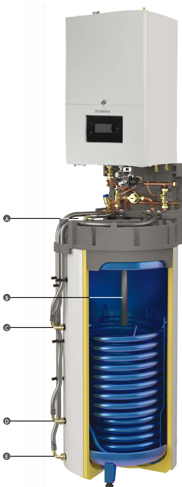
A Sortie eau chaude sanitaire du préparateur B Anode en magnésium C Entrée échangeur
