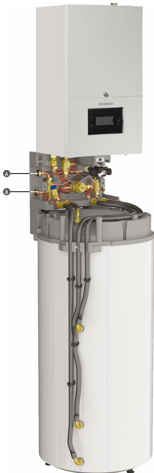
A Entrée eau froide sanitaire B Sortie eau chaude sanitaire
