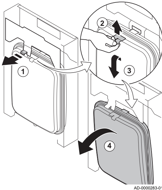
Fig.88 Dépose du vase d'expansion
