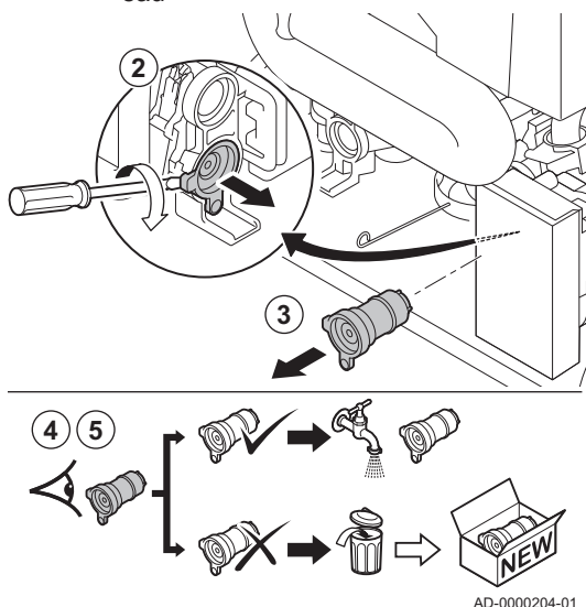
Fig.83 Nettoyage de la cartouche filtre à eau
