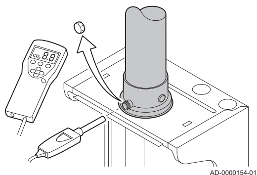
Fig.65 Prise de mesure des fumées
