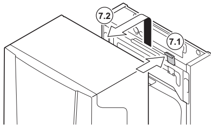
Fig.87 Dépose de la partie avant de la chaudière
