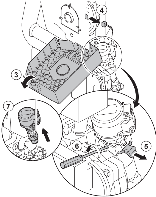
Fig.79 Remplacement de la vanne 3 voies
