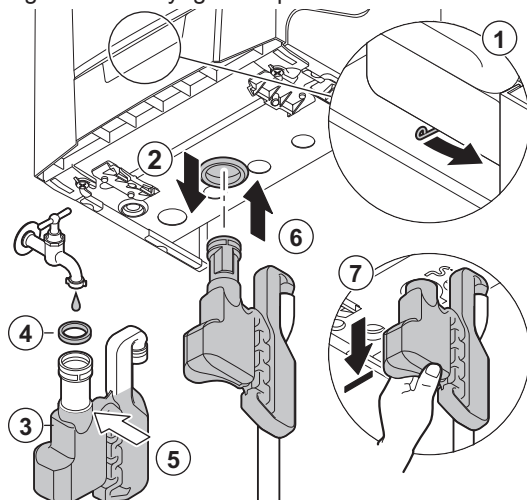
Fig.72 Nettoyage du siphon
