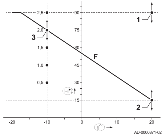
Fig.35 Courbe de chauffe interne
