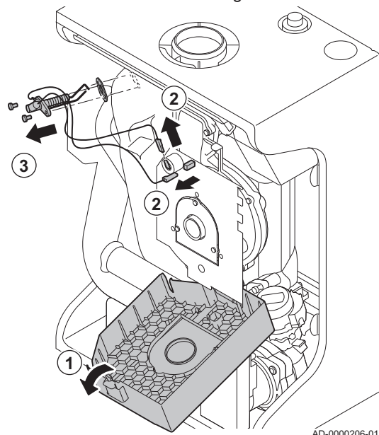
Fig.77 Remplacement de l'électrode d'ionisation/d'allumage
