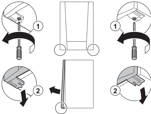
Fig.58 Ouverture de la chaudière
