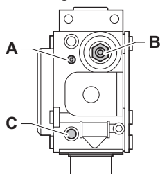
Fig.70 Bloc vanne gaz
