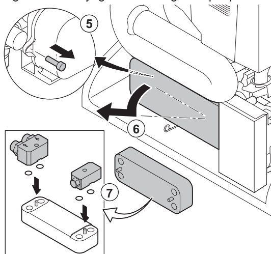
Fig.82 Nettoyage de l'échangeur à plaques
