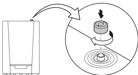
Fig.71 Contrôle du purgeur automatique
